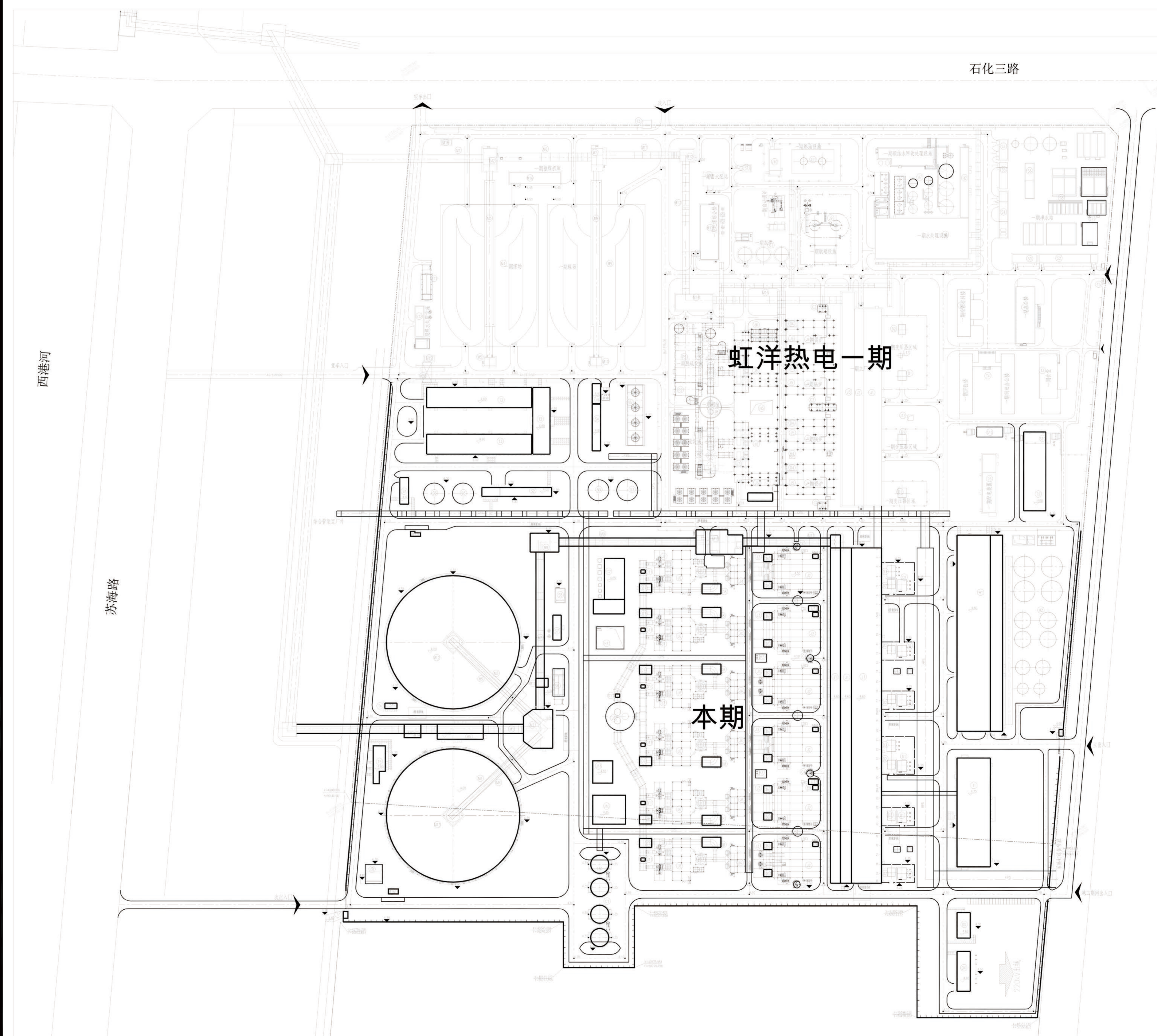
总平面布置图 1:1000
